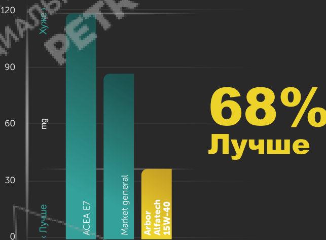
ЗАЩИТА ОТ ИЗНОСА потеря массы на верхнем поршневом кольце Mack T-12
